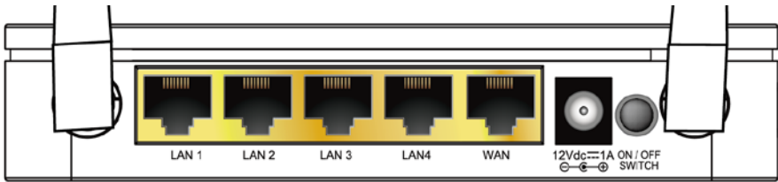
Figuur 1: Aansluitingen router achterzijde
